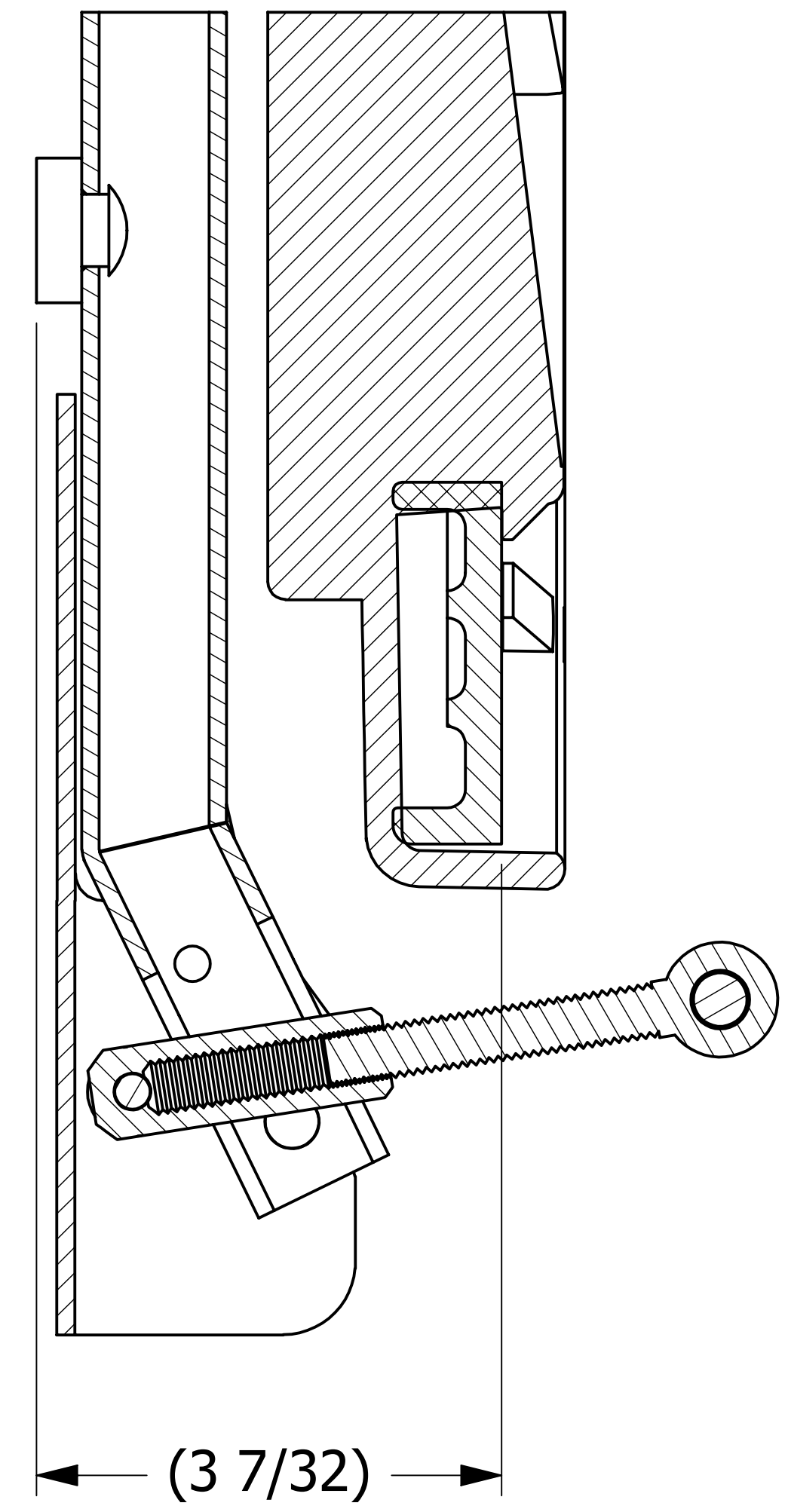
SECTION A-A SCALE 1:1
